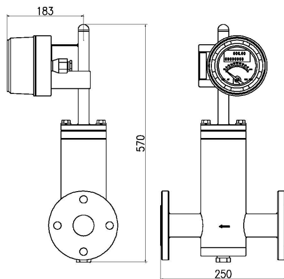
图 7 T 型结构 M5 指示器
