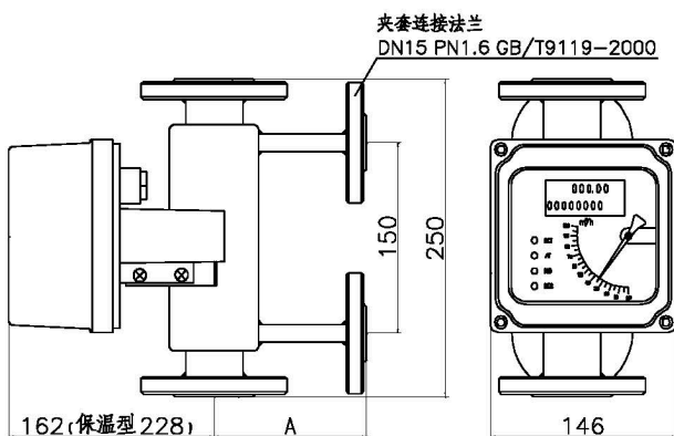
图4 冷却夹套型 M4 指示器
