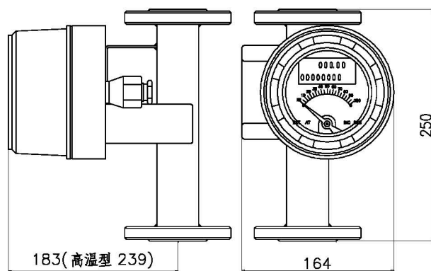
图3 标准型 M5 指示器
