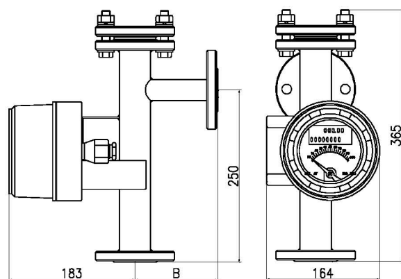
图 11 标准型 M5 指示器
