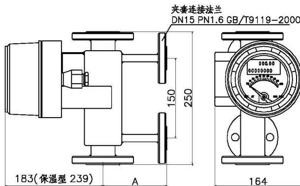
图5 冷却夹套型 M5 指示器
