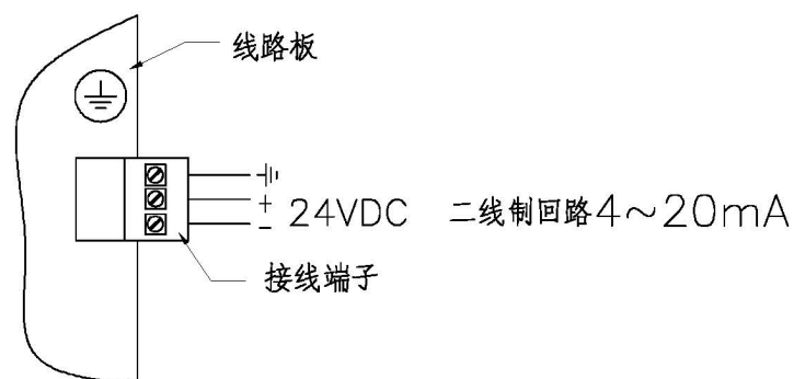
圆表壳
