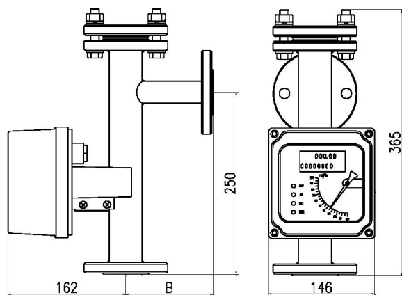
图 10 标准型 M4 指示器
